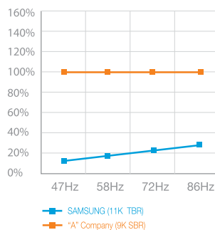
Тест уровня вибрации (ASHRAE) Компрессор BLDC (двойной ротор)
